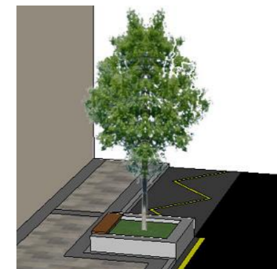
DETALLE ALCORQUE DE GRANITO CON ASIENTO EN MADERA
