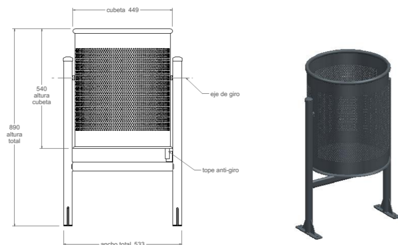
DETALLE PAPELERA CIRCULAR DE CHAPA DE ACERO
