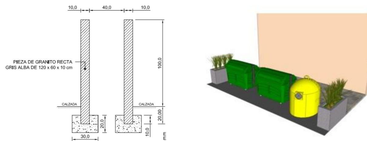
SECCIÓN JARDINERA RECTA OCULTA CONTENEDORES
